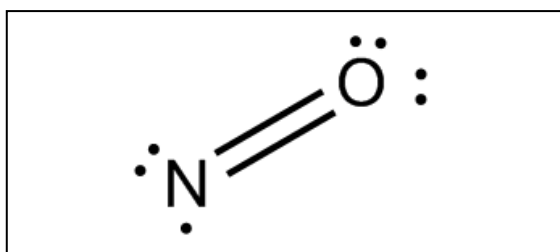
Figur 1. Strukturformel av nitrogenmonoksid.
